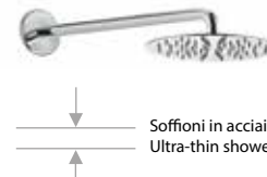
30CR8630 Soffione Ø200 mm con braccio 350 mm. Shower head Ø200 mm with inlet arm 350 mm.
